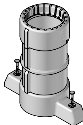
斜視図
